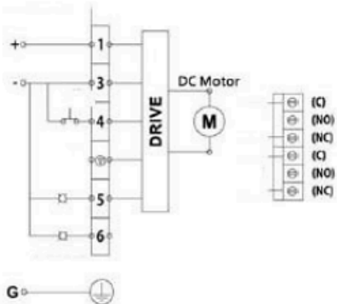
VSE-1-S~VSE-12 DC24V
