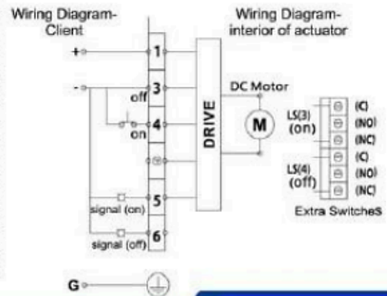
VSE-1-S~VSE-12 DC24V WIRING DIAGRAM
