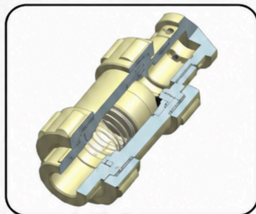
Corte interno
