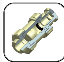
Corte interno
